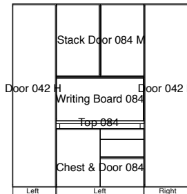
Door 042 H (L) + Stack door 084 M + Writing Board 084 + Top 084 + Chest & Door 084 (L) + Door 042 H (R) W168. D44. H182 (oak, walnut)
