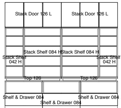
Stack Door 126 L + Stack Door 126 L + Stack Shelf 042 H + Stack Shelf 084 H + Stack Shelf 084 H + Stack Shelf 042 H + Top 126 + Top 126 + Shelf & Drawer 084 + Shelf & Drawer 084 + Shelf & Drawer 084 W252. D44. H238
