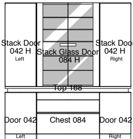
Stack Door 042 H (L) + Stack Glass Door 084 H + Stack Door 042 H (R) + Top 168 + Door 042 (L) + Chest 084 + Door 042 (R) W168, D44, H182
