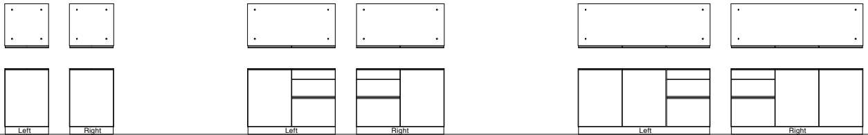
Door 042 (L), (R) W42. D42. H63 (oak,walnut) (Black) Chest & Door 084 (L), (R) W84. D42. H63 (oak,walnut) (Black) Chest & Door 126 (L), (R) W126. D42. H63 (oak,walnut) (Black)
