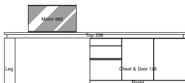
Top 238 + Leg + Chest & Door 126 (R) W238. D44. H70
