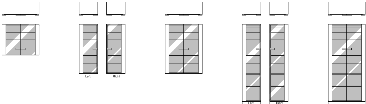
Stack Glass Door 084 M W84, D30, H70
