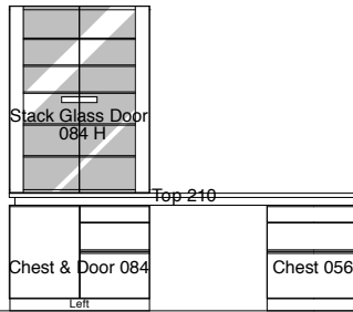
Stack Glass Door 084 H + Top 210 + Chest & Door 084 (L) + Chest 056 W210. D44. H182
