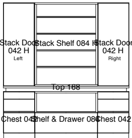
Stack Door 042 H (L) + Stack Shelf 084 H + Stack Door 042 H (R) + Top 168 + Chest 042 + Shelf & Drawer 084 + Chest 042 W168, D44, H182
