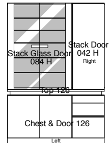
Stack Glass Door 084 H + Stack Door 042 H (R) + Top 126 + Chest & Door 126 (L) W126, D44, H182
