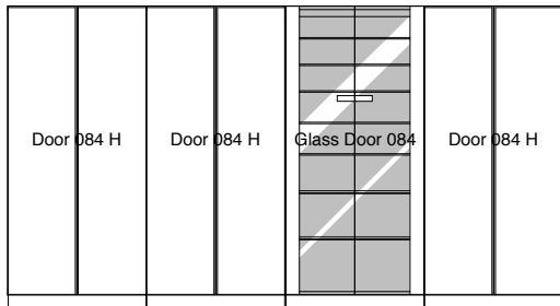
Door 084 H + Door 084 H + Glass Door 084 H + Door 084 H W336. D30. H182 (oak, walnut)
