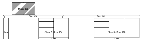
Top 168 + Top 210 + Leg + Chest & Door 084(L) + Chest & Door 126 (L) W378. D44. H70
