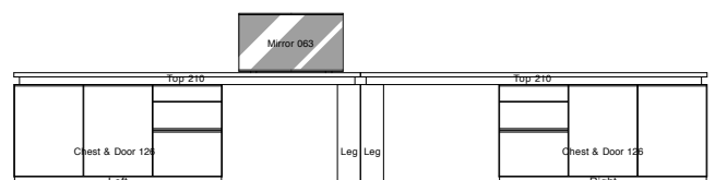
Top 210 + Top 210 + Chest & Door 126 (L) + Leg + Leg + Chest & Door 126 (R) W420. D44. H70
