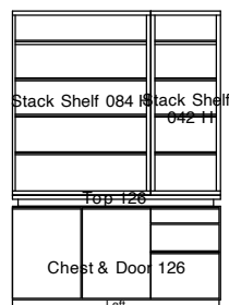
Stack Shelf 084 H + Stack Shelf 042 H + Top 126 + Chest & Door 126 (L) W126. D44. H182
