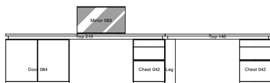
Top 210 + Top 140 + Door 084 + Chest 042 + Leg + Chest 042 W350. D44. H70
