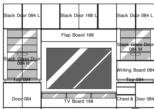
Stack Door 084 L + Stack Door 168 L + Stack Door 084 L + Stack Glass Door 084 H + Flap Board 168 + Stack Glass Door 084 M + Writing Board 084 + Top 084 + Top 084 + Door 084 + TV Board 168 + Chest & Door 084 (R) W336. D56. H238
