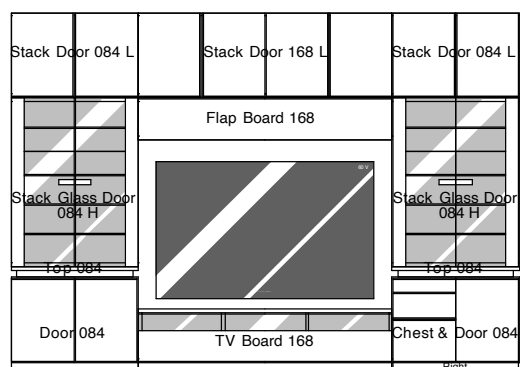
Stack Door 084 L + Stack Door 168 L + Stack Door 084 L + Stack Glass Door 084 H + Flap Board 168 + Stack Glass Door 084 H + Top 084 + Top 084 + Door 084 + TV Board 168 + Chest & Door 084 (R) W336. D56. H238
