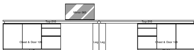
Top 210 + Top 210 + Chest + Door 126 (L) + Leg + Leg + Chest + Door 126 (R) W420. D44. H70
