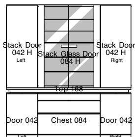
Stack Door 042 H (L) + Stack Glass Door 084 H + Stack Door 042 H (R) + Top 168 + Door 042 (L) + Chest 084 + Door 042 (R) W168. D44. H182
