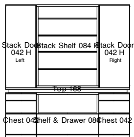
Stack Door 042 H (L) + Stack Shelf 084 H + Stack Door 042 H (R) + Top 168 + Chest 042 + Shelf & Drawer 084 + Chest 042 W168. D44. H182
